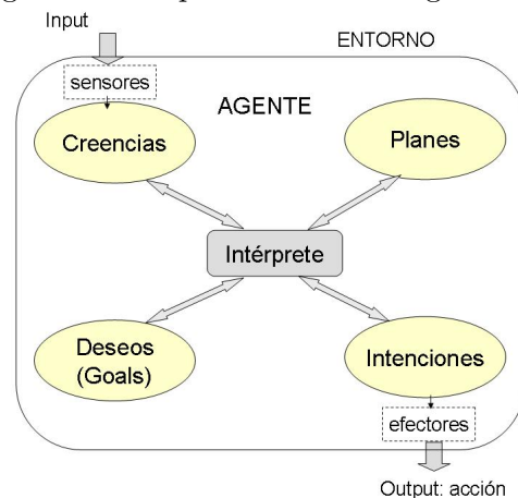
Figura 4.2: Arquitectura de un agente PRS
