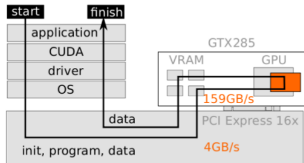
Figura 9.4: (secuencial) + GPU (paralelo) (Pospichal, Jaros, & Schwarz, 2010)
