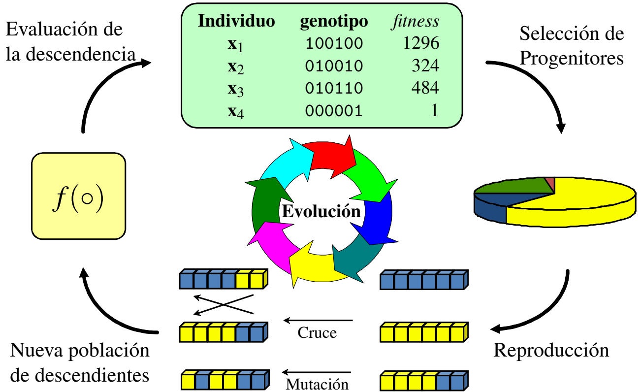
Figura 7.6: Ciclo principal de un Algoritmo Genético
