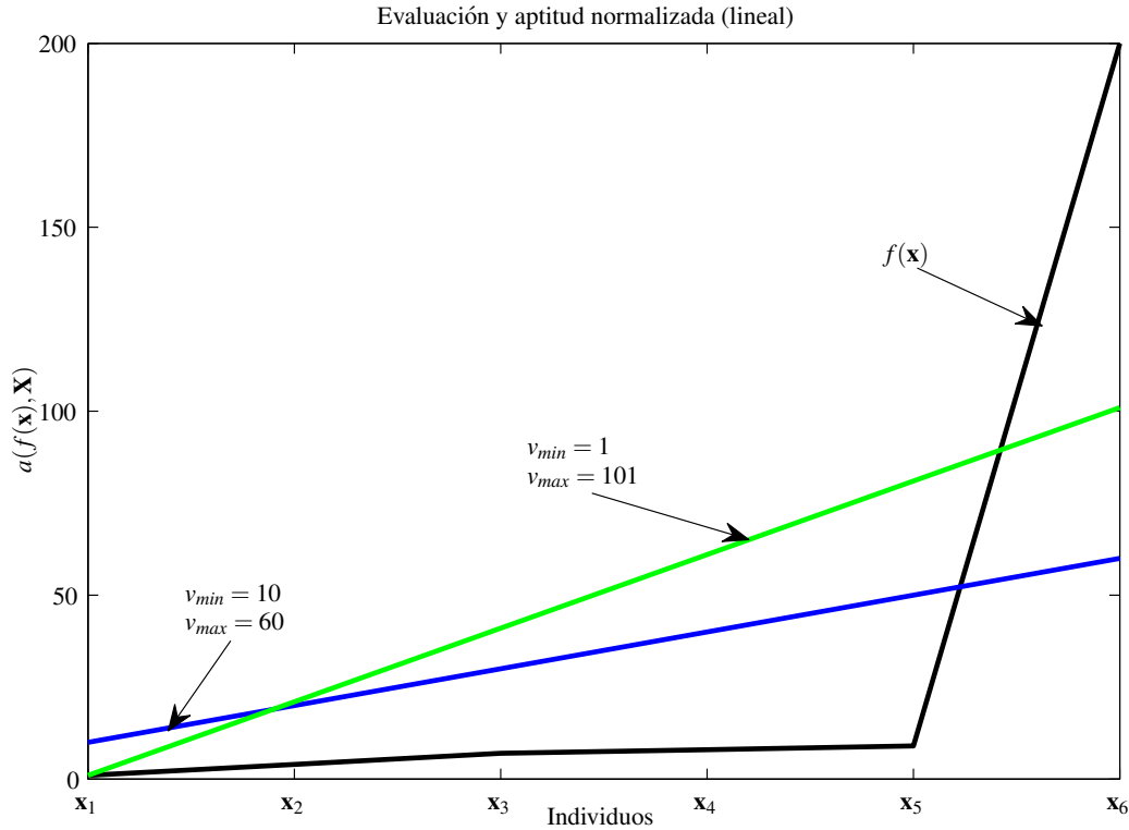
Figura 7.15: Ejemplo de Normalización lineal
