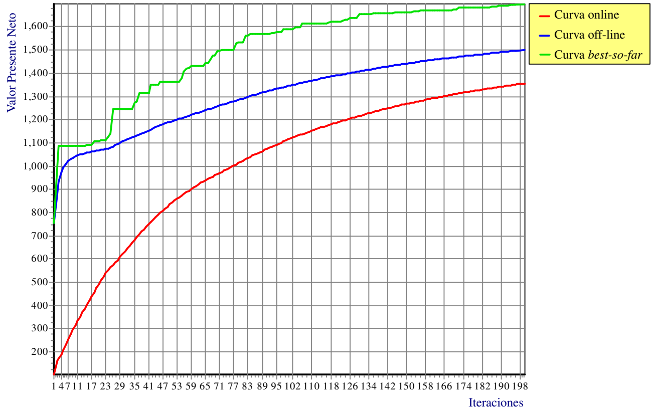
Figura 7.17: Ejemplo de curvas best-so-far , off-line y online .
