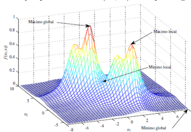
Figura 6.1: Ejemplo de función f(x_1, x_2) con óptimo global y local
