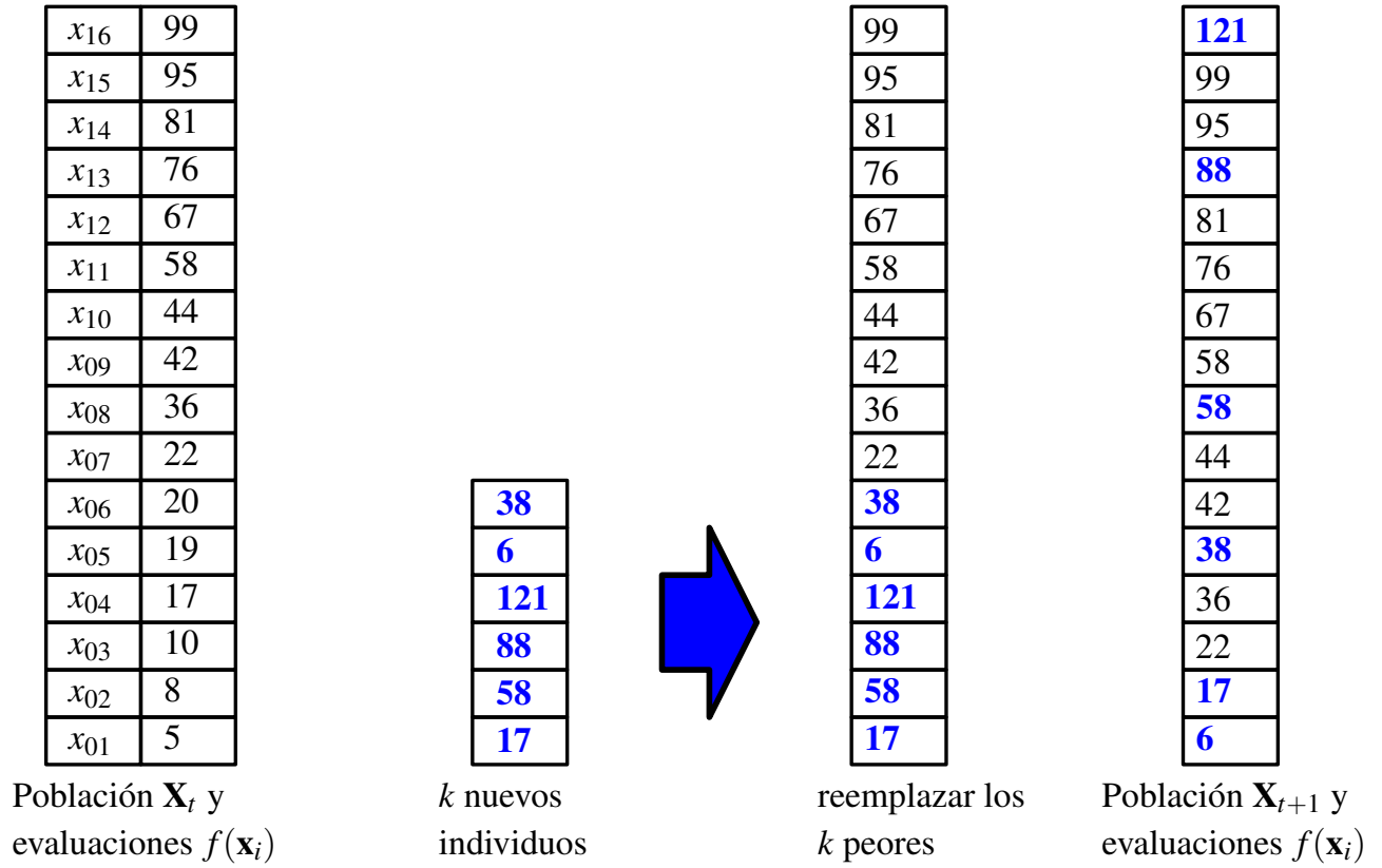
Figura 7.16: Procedimiento Steady-state
