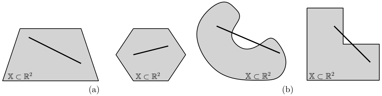
Figura 7.2: Espacios convexos y no convexos
