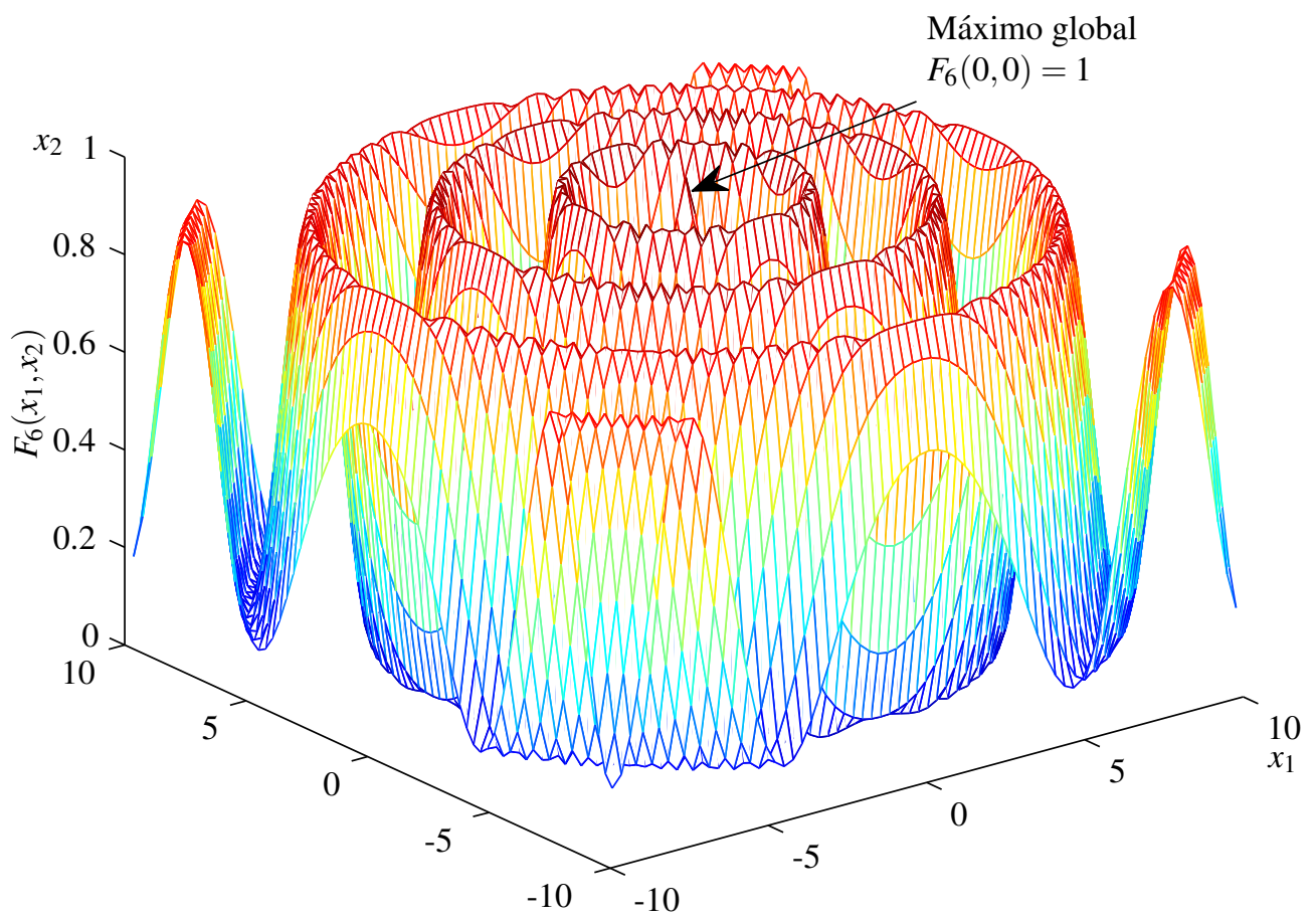
Figura 7.8: Visualización de la Función F_6
