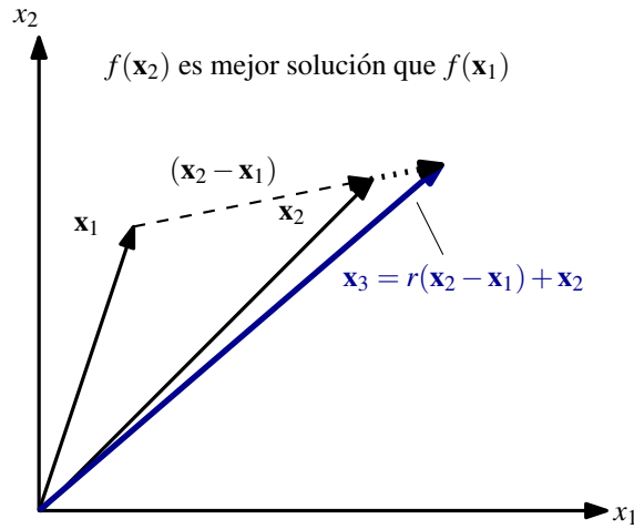
Figura 7.20: Cruce Heurístico
