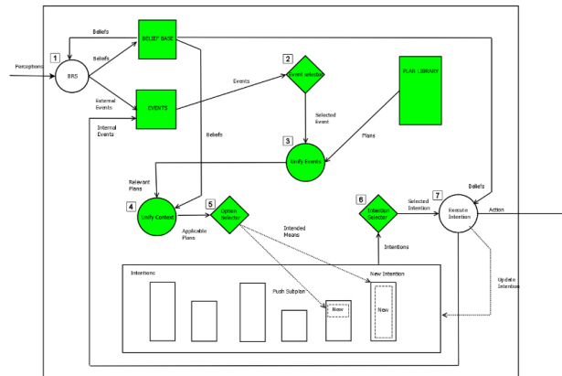
Figura 4.3: Máquina de estados de un agente PRS (Bordini &amp; Hübner, 2007)
