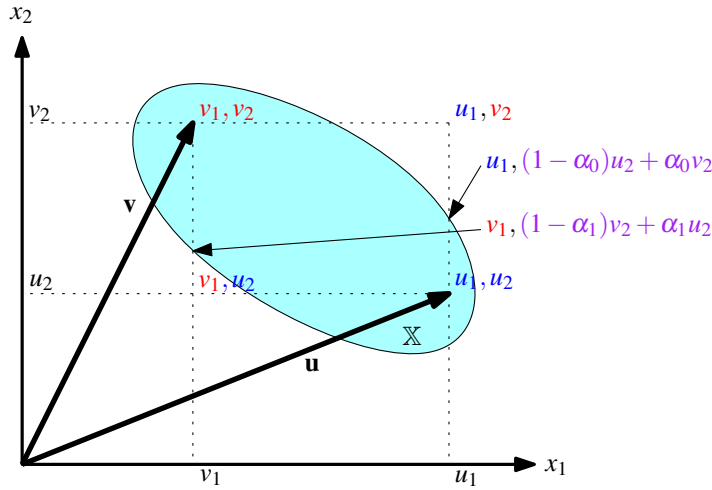
Figura 7.19: Cruce Simple
