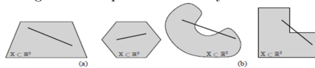
Figura 6.2: Espacios convexos y no convexos
