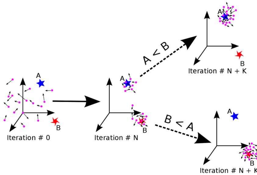
Figura 8.10: Comportamiento del PSO
