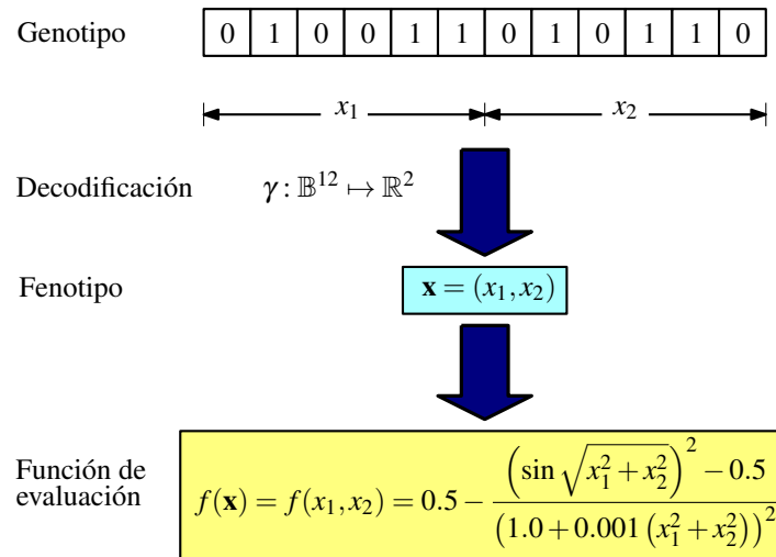
Figura 7.9: Cromosoma y Función de Evaluación
