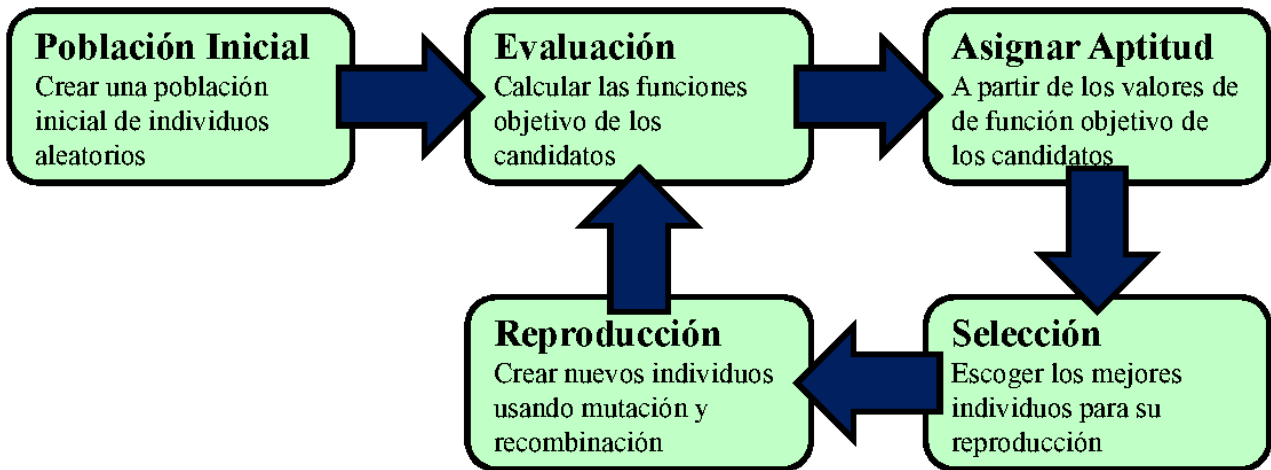
Figura 7.3: El ciclo básico de un Algoritmo Evolutivo
