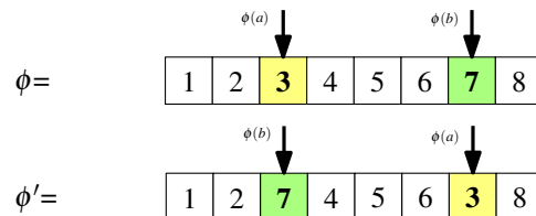
Figura 7.26: Ejemplo de mutación basada en posición
