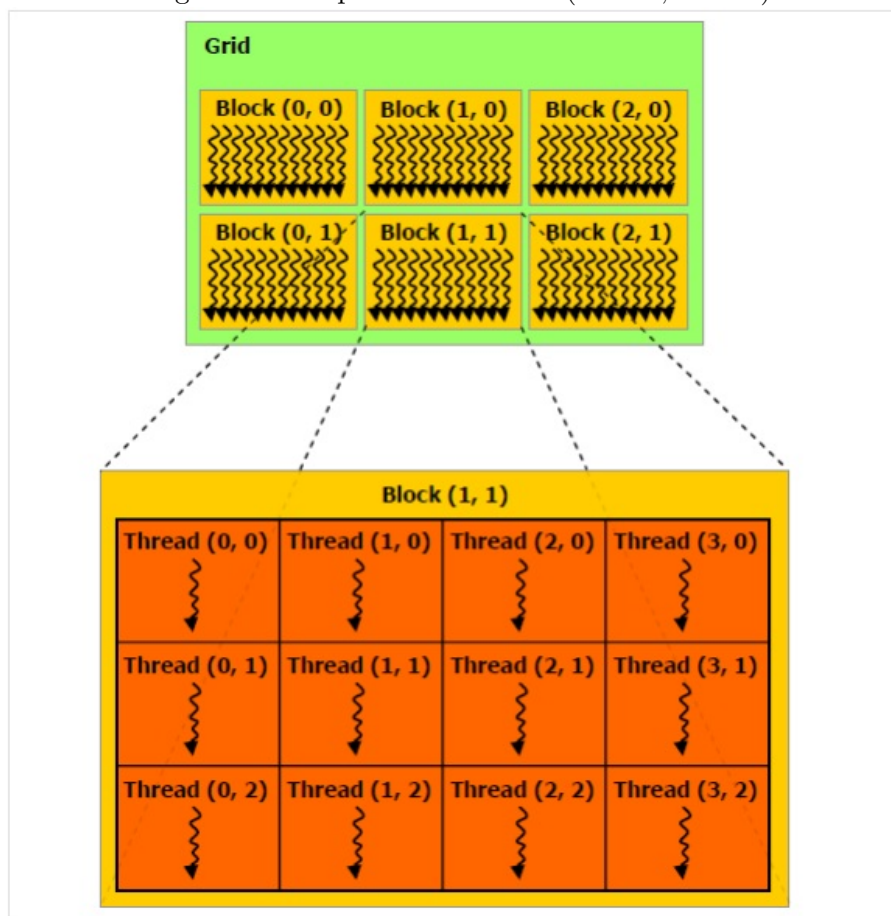
Figura 9.2: Arquitectura CUDA (Nvidia, 2011 a)
