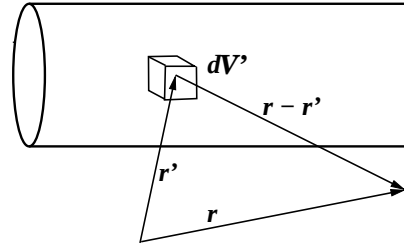
Figura 4.2: Se considera un elemento de volumen dV' en el conductor con corriente. Este pequeño volumen es responsable de una parte d^3\vec{B} del campo total que la corriente provoca y está dada en (4.1.6).
