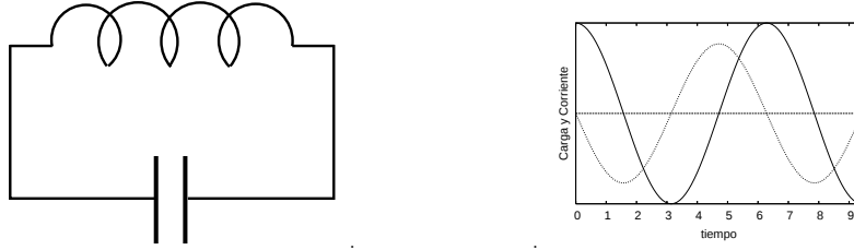
Figura 6.10: Izquierda: Un circuito ideal LC: la diferencia de potencial en el condensador debe ser igual a la fem autoinducida en la bobina. Derecha: la carga Q(t) (medida en Coulomb) representada por la línea continua y la corriente I(t) (medida en Ampère) en línea de puntos.
