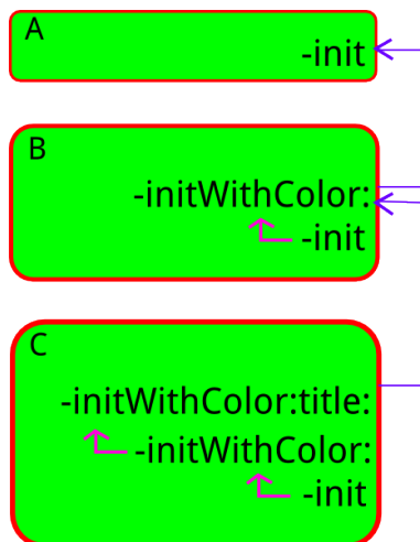
Figura 6-1. Jerarquía de los métodos de inicio.
