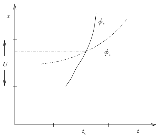
Figura 4.3: Prueba de la unicidad de la solución.
