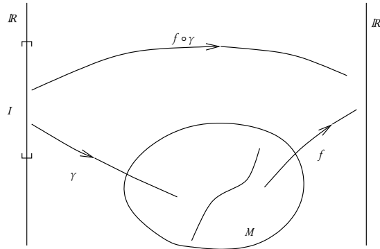
Figura 3.8: Definición de vector.
