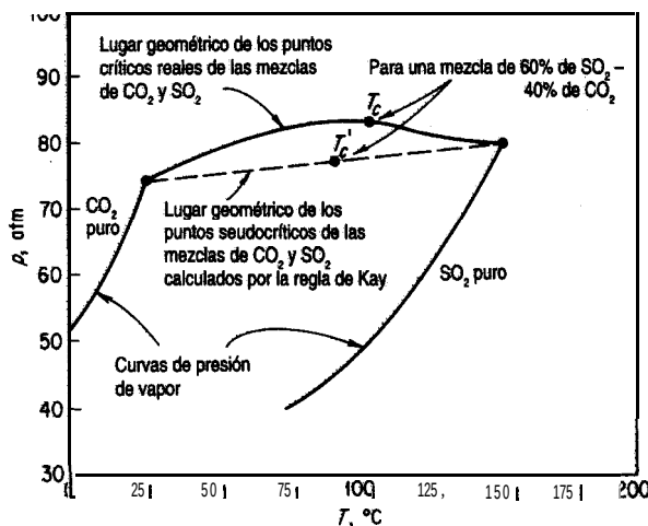
Figura 4.9 Puntos crítico y seudocrítico para una mezcla de CO, y SO 2 .
