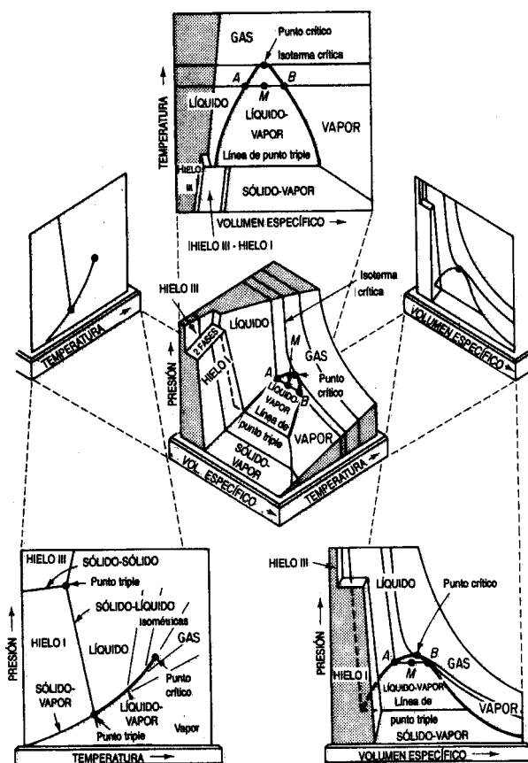
Figura 4.10 Superficie p - \hat{V} - T y proyecciones para H_2O .
