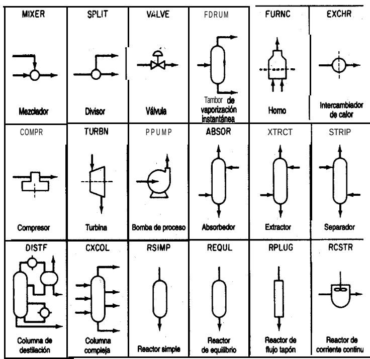
Figura 6.11 Módulos de proceso típicos empleados en los programas de simulación secuencial basados en módulos, junto con los nombres de sus subrutinas.
