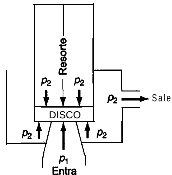
(B) Esta válvula tiene las partes inferior y superior del disco de cierre abiertas a la salida ( p_2 )
