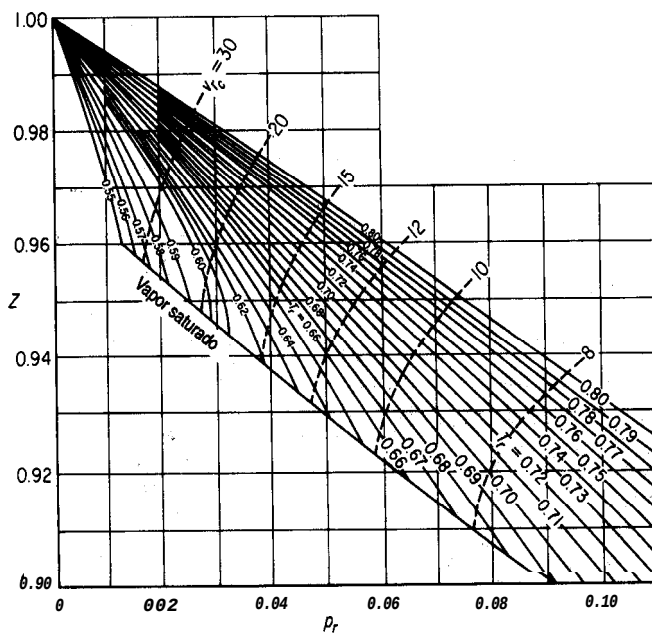
Figura 4.5 a) Carta de compresibilidad generalizada que muestra las porciones respectivas de las cartas expandidas subsecuentes. b) Carta de compresibilidad generalizada, presión reducida muy baja. c) Carta de compresibilidad generalizada, baja presión. d) Carta de compresibilidad generalizada, presiones medianas. e) Carta de compresibilidad generalizada, presiones altas.
