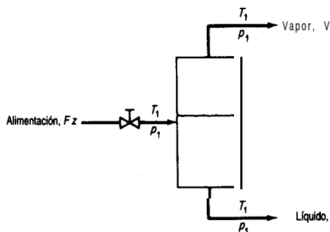
Figura 6.14 Separador vapor-líquido
