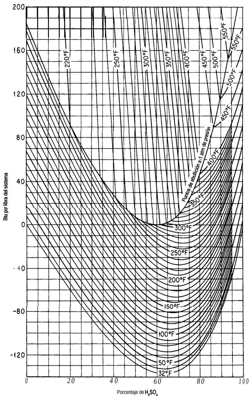
Figura 1.4 Diagrama de entalpía-concentración del sistema ácido sulfúrico-agua relativo a los componentes puros. (Agua y \text{H}_2\text{SO}_4 a 32^\circ\text{F} y su propia presión de vapor.) (Datos de International Critical Tables , © 1943 O. A. Hougen y K. M. Watson.)
