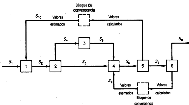
Figura 6.15 Secuencia de computación para programas de simulación modular. Se estiman los valores iniciales de ambas recirculaciones y luego se resuelven los módulos en el orden 1, 2, 3, 4, 5 y 6. Los valores calculados para las corrientes de recirculación S_9 y S_{10} se comparan con los valores estimados dentro de un bloque de convergencia y, a menos que la diferencia sea menor que cierta tolerancia prescrita, se realiza otra iteración con los valores calculados, o con estimaciones basadas en ellos, formando los nuevos valores estimados iniciales de las corrientes de recirculación.
