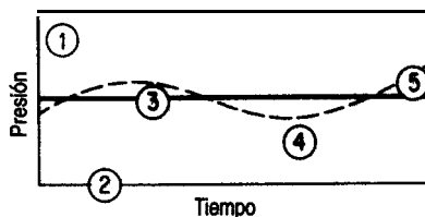
Figura 1.12 Terminología de presión. La atmósfera estándar se indica con la línea horizontal gruesa. La línea interrumpida ilustra la presión atmosférica (barométrica) que cambia con el tiempo. El punto ① de la figura corresponde a una presión de 19.3 psi referida a un vacío completo, o de 5 psi referida a la presión barométrica; ②, es el vacío completo; ③ representa la atmósfera estándar, y ④ ilustra una presión relativa negativa o una presión menor que la atmosférica. Este tipo de medición se describe en el texto como una medición de vacío. El punto ⑤ también indica una medición de vacío, pero ésta equivale a una presión absoluta superior a la atmósfera estándar .
