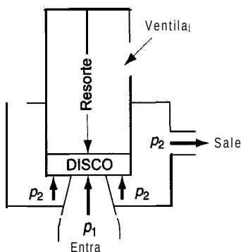
(A) Esta válvula tiene la parte superior del disco de cierre abierta a la salida ( p_2 )
