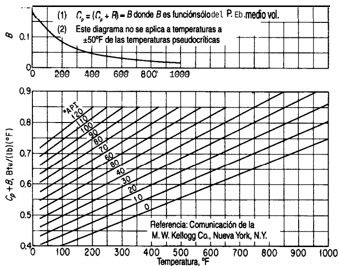
Figura K.1 Calores específicos de hidrocarburos líquidos.
