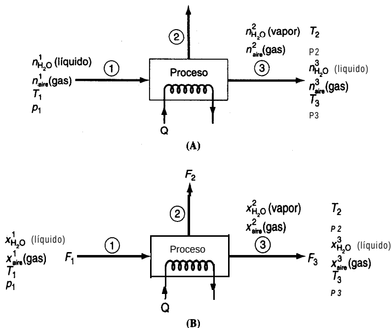
Figura 6.2 Proceso sencillo con tres flujos en el que (A) los flujos de las corrientes se expresan como velocidades de flujo molar; y (B) el flujo de la corriente es el flujo total y las composiciones de las especies se indican en fracciones molares.
