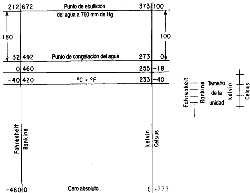
Figura 1.5 Escalas de temperatura.
