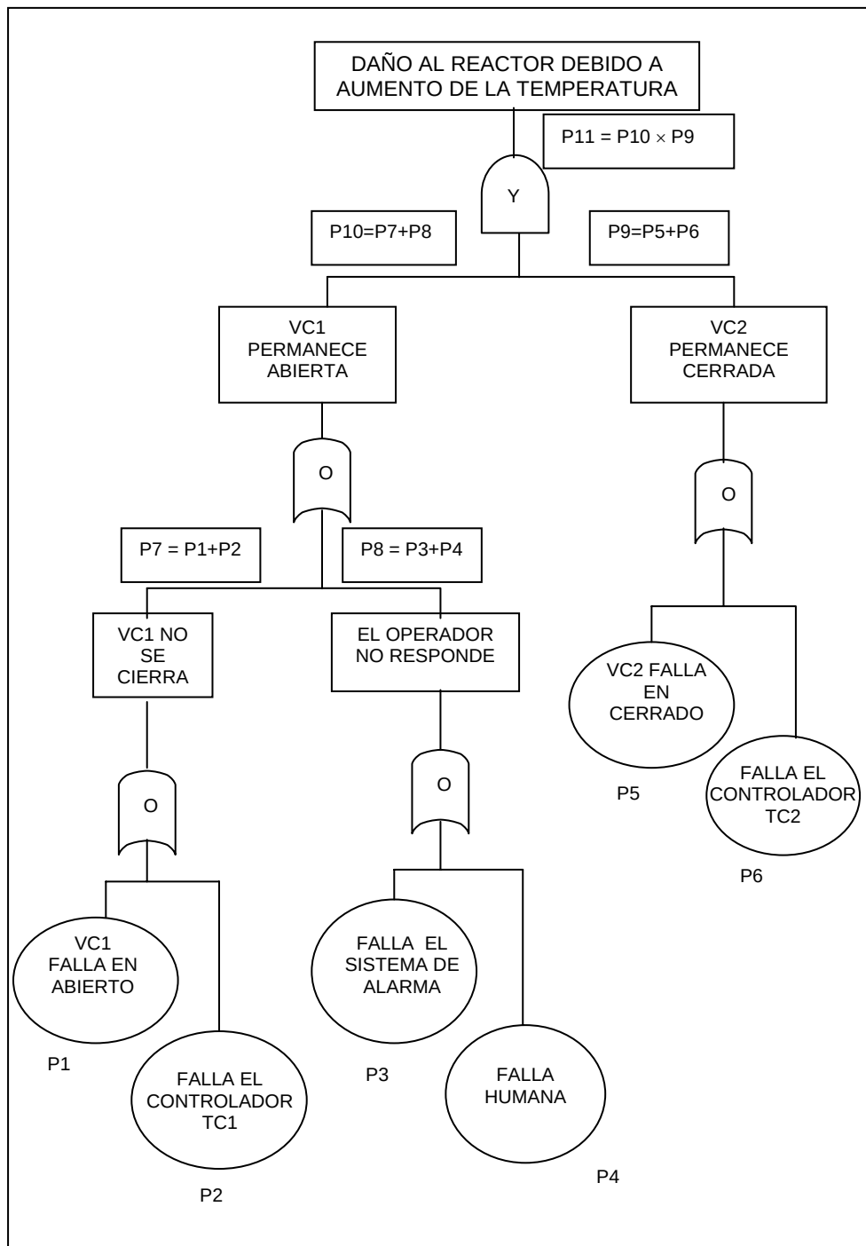
FIGURA 11.8: ÁRBOL DE FALLA PARA REACTOR DE LA FIGURA 11.5
