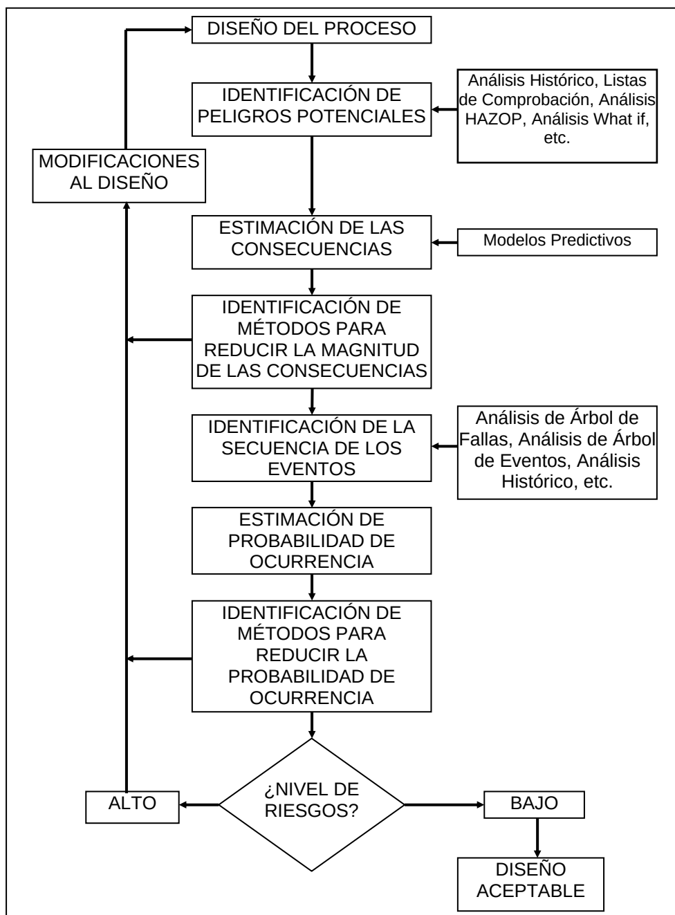
FIGURA 11.1: ETAPAS TÍPICAS DE UN ANÁLISIS DE RIESGO EN EL CONTEXTO DEL DISEÑO DE PROCESOS MÁS SEGUROS
