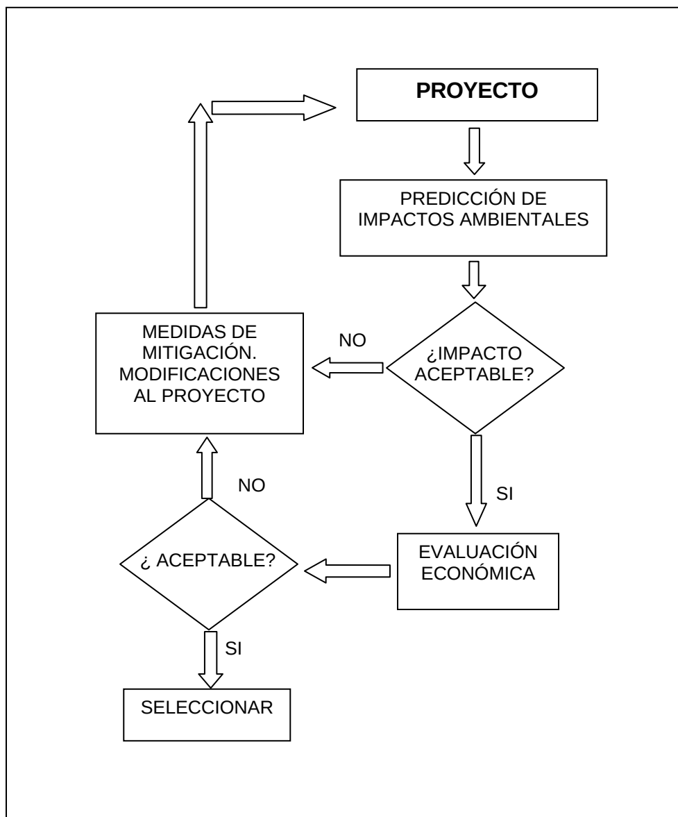
FIGURA 6.3: DISEÑO DE PROCESOS LIMPIOS
