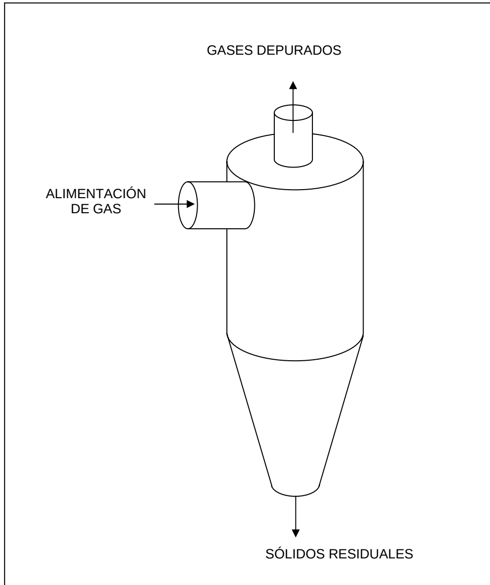
FIGURA 5.8: CICLÓN PARA ELIMINACIÓN DE MATERIAL PARTICULADO EN GASES
