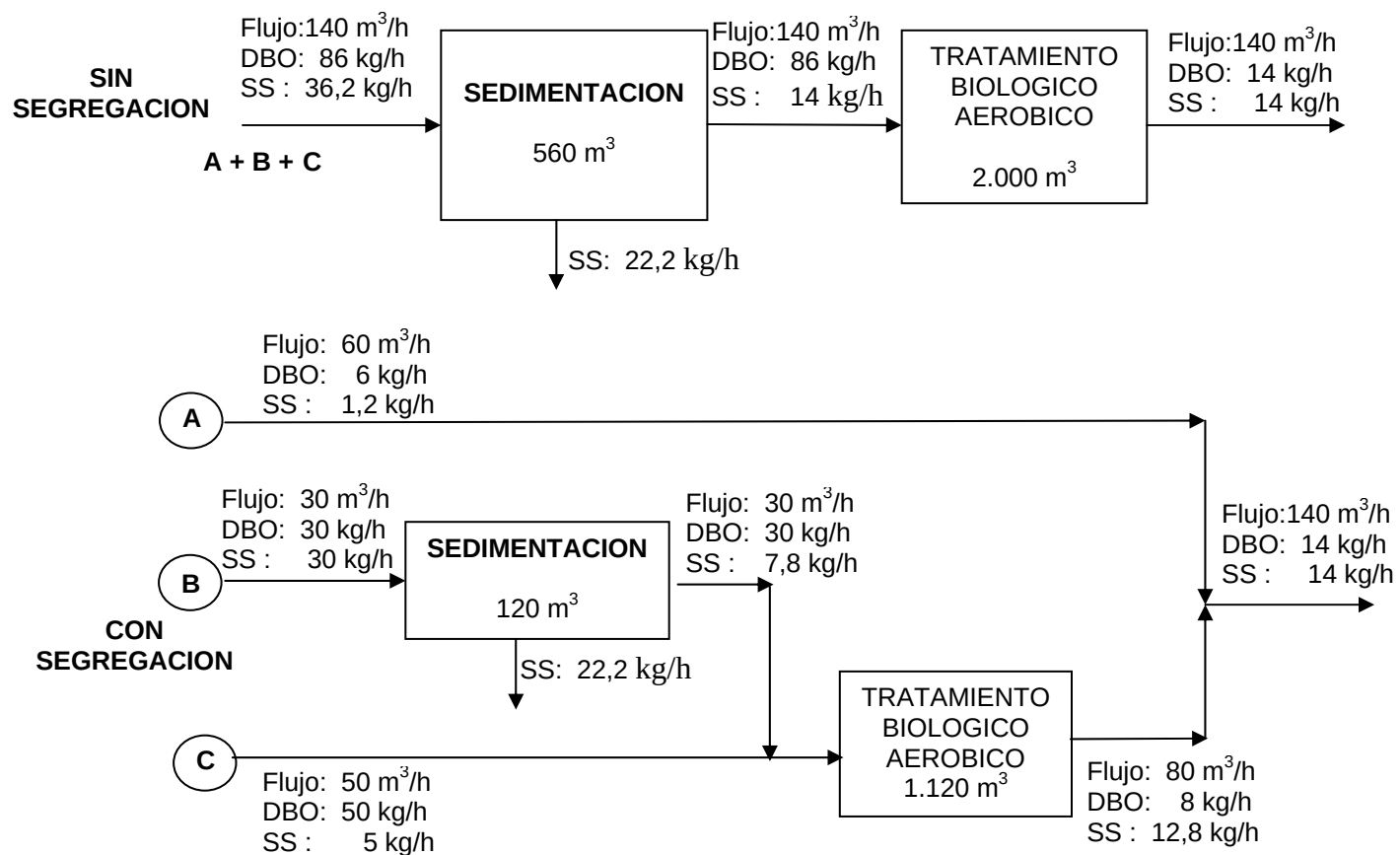
FIGURA 6.6: TRATAMIENTO DIFERENCIADO DE EFLUENTES SEGREGADOS
