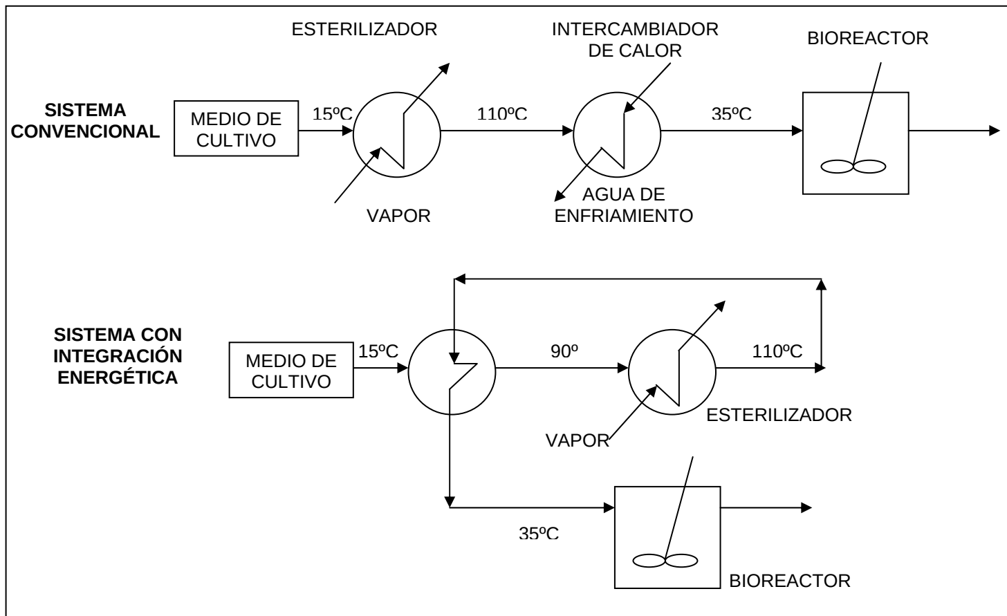
FIGURA 6.8: INTEGRACIÓN ENERGÉTICA EN UN SISTEMA DE FERMENTACIÓN INDUSTRIAL
