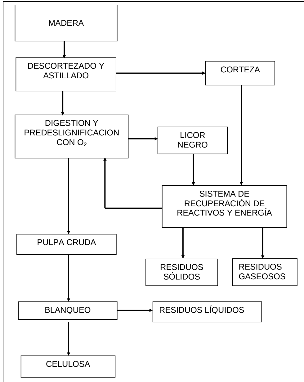
FIGURA 4.6: PRODUCCIÓN DE CELULOSA BLANCA. PROCESO KRAFT
