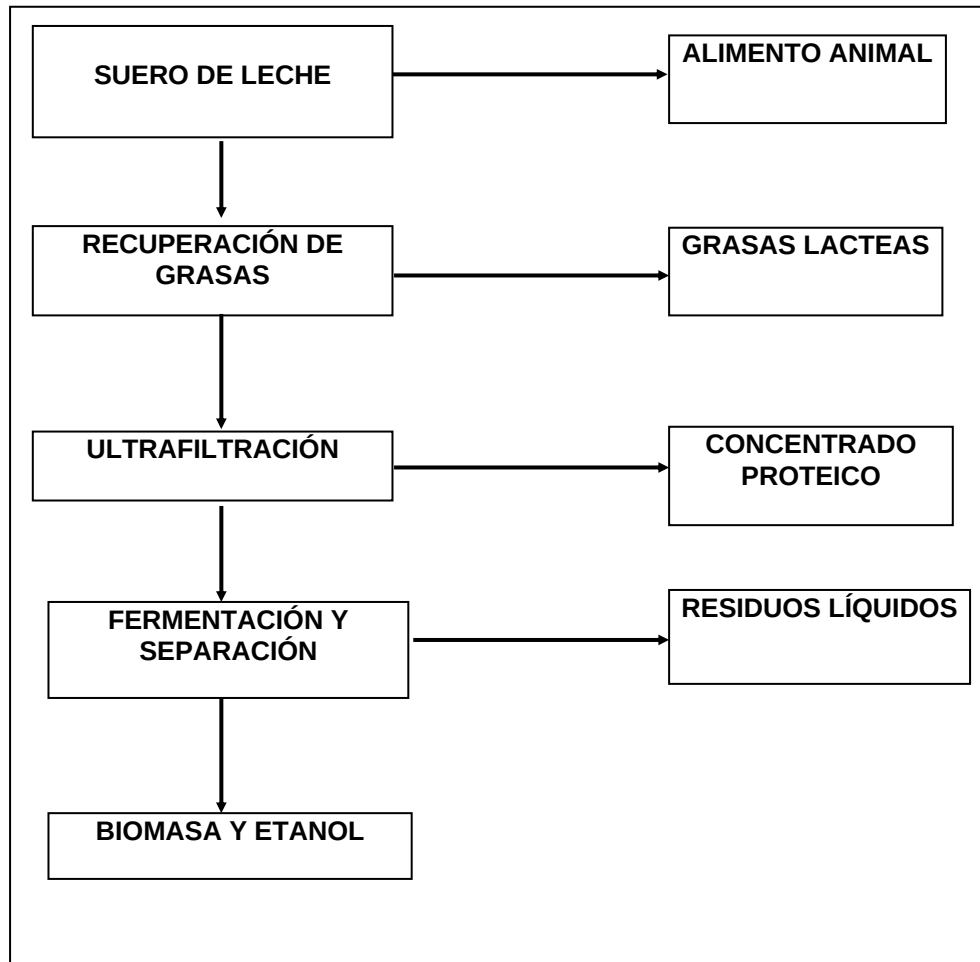
FIGURA 4.2: PROCESAMIENTO DEL SUERO DE LA LECHE
