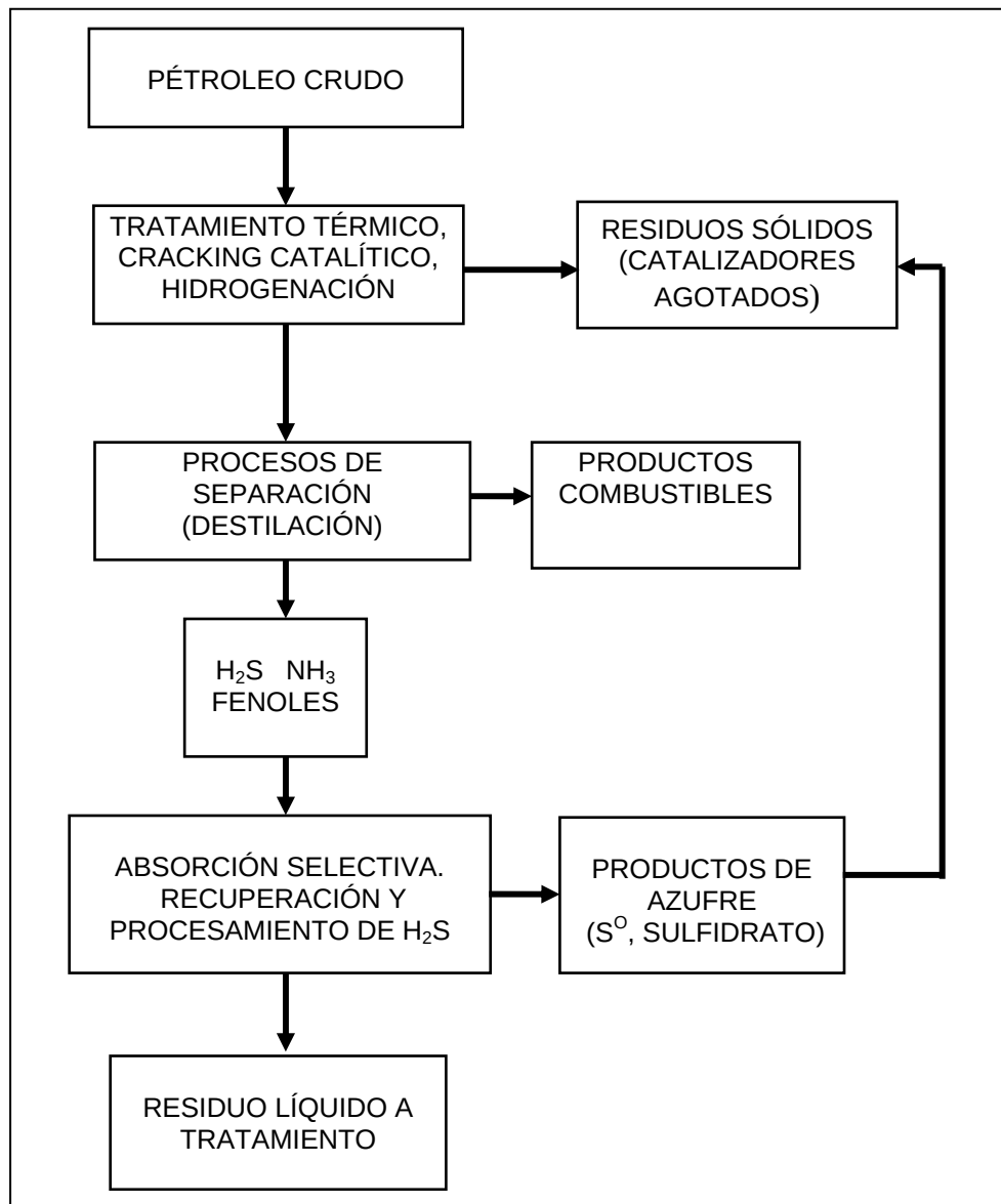
FIGURA 4.7: REFINACIÓN DEL PÉTROLEO
