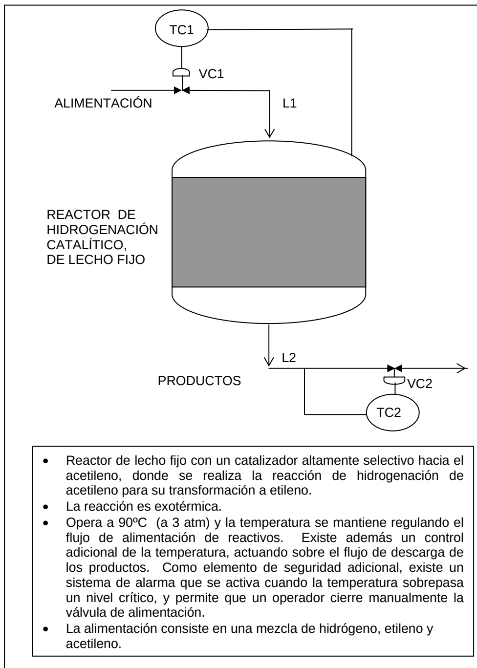
FIGURA 11.5: HIDROGENACIÓN CATALÍTICA DE ACETILENO
