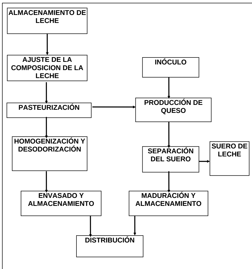
FIGURA 4.1: PRODUCCIÓN DE LECHE Y QUESO
