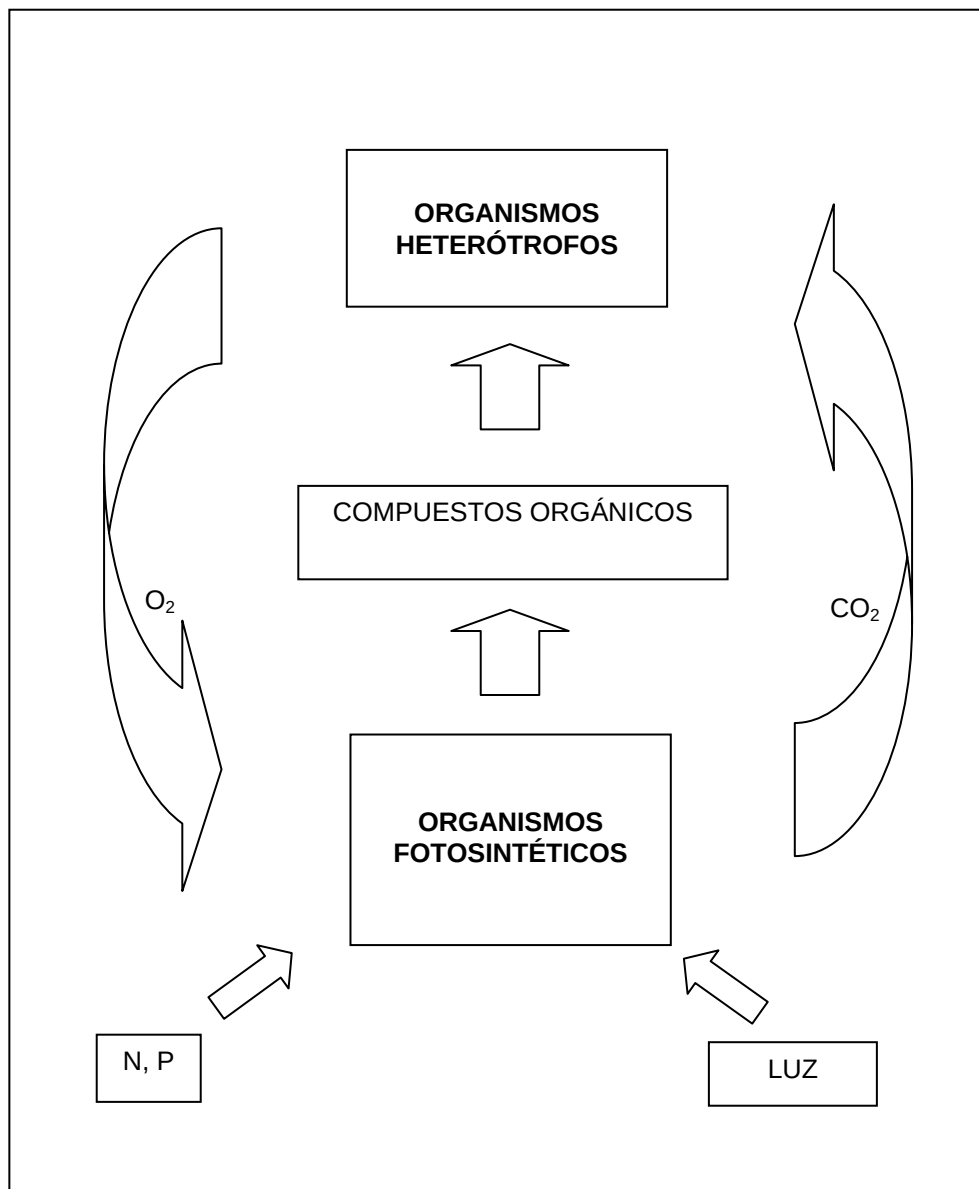
FIGURA 3.8: CADENA TRÓFICA SIMPLIFICADA
