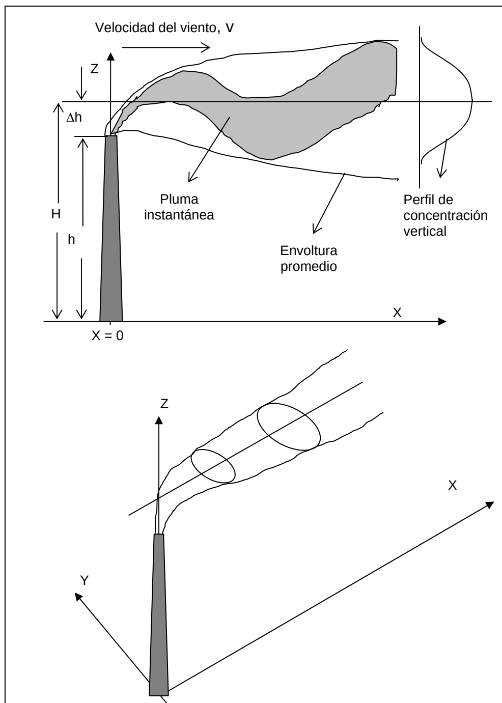
FIGURA 3.6: PRESENTA LA CHIMENEA SITUADA EN EL ORIGEN, CON EL VIENTO EN LA DIRECCIÓN X.
