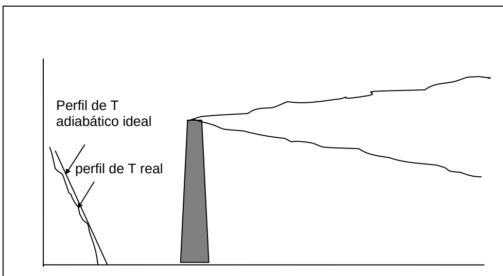
FIGURA 3.3: DISPERSIÓN EN FORMA DE CONO. PERFIL DE TEMPERATURA SIMILAR AL PERFIL ADIABÁTICO IDEAL. ATMÓSFERA LEVEMENTE INESTABLE. LLEGA AL SUELO A MAYOR DISTANCIA.
