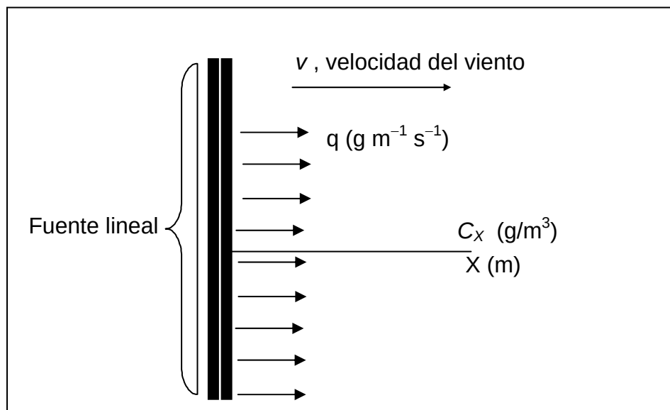
FIGURA 3.7: MODELACIÓN DEL EFECTO DE FUENTES CONTAMINANTES ATMOSFÉRICOS DE TIPO LINEAL.
