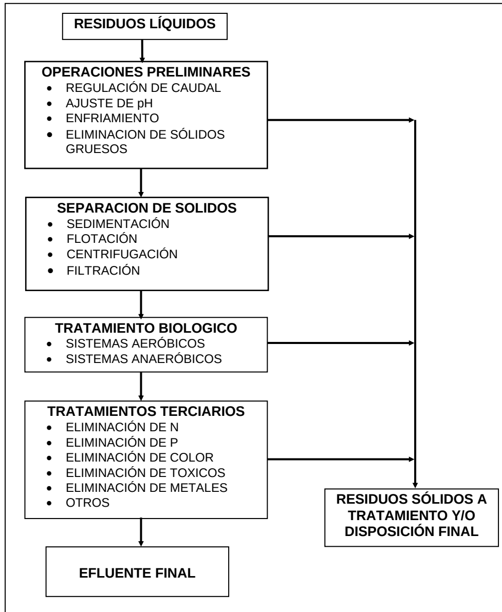
FIGURA 5.1: SISTEMA TÍPICO PARA EL TRATAMIENTO DE RESIDUOS LÍQUIDOS
