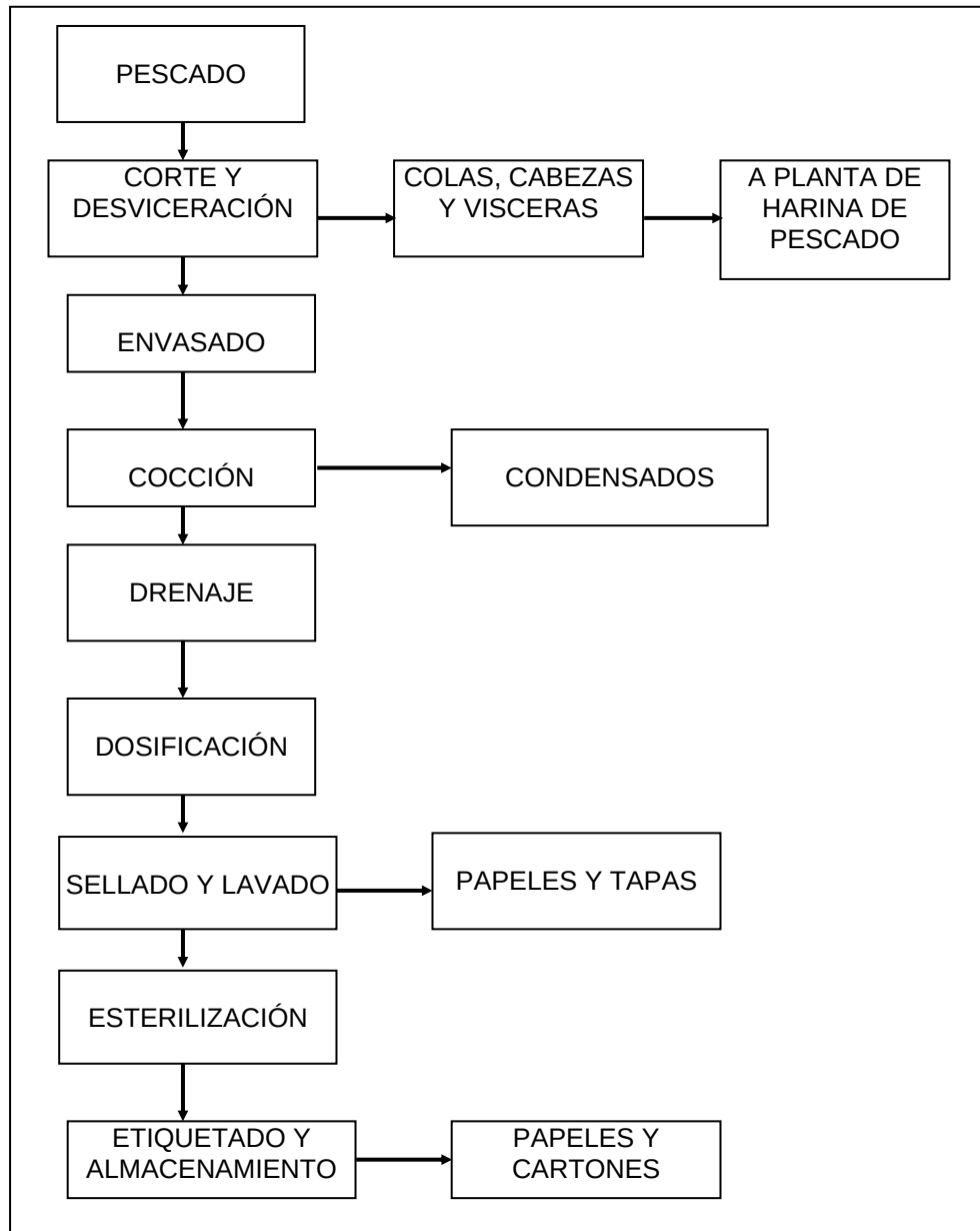
FIGURA 4.4: ELABORACIÓN DE CONSERVAS
