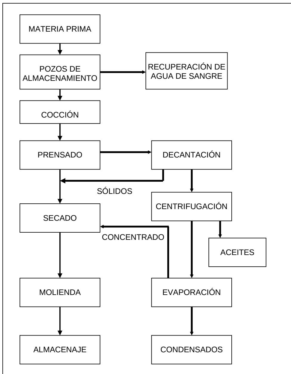
FIGURA 4.5: ELABORACIÓN DE HARINA Y ACEITE DE PESCADO
