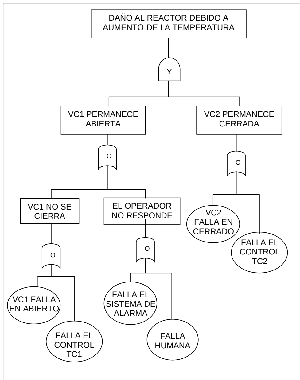
FIGURA 11.6: ÁRBOL DE FALLA PARA REACTOR DE LA FIGURA 11.5
