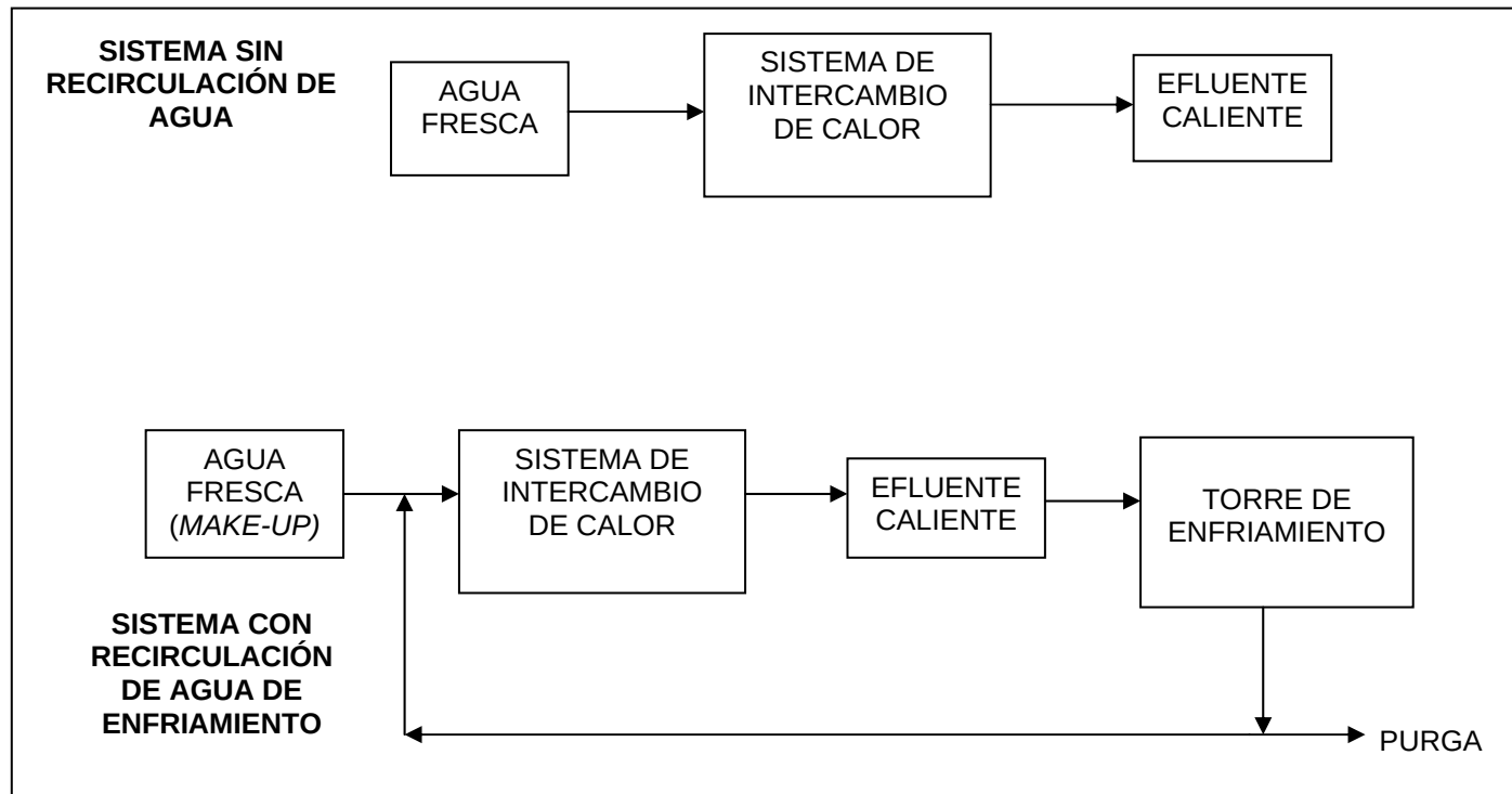
FIGURA 6.9: SISTEMA DE INTERCAMBIO DE CALOR SIN Y CON RECIRCULACIÓN DE AGUA DE ENFRIAMIENTO
