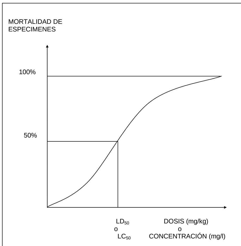
FIGURA 3.15: RELACIÓN DOSIS – RESPUESTA . ENSAYOS DE TOXICIDAD AGUDA.
