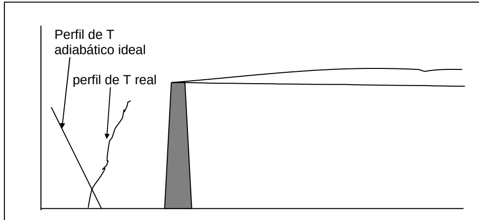
FIGURA 3.4: DISPERSIÓN EN FORMA DE ABANICO. PERFIL DE TEMPERATURA INVERTIDO. ATMÓSFERA ESTABLE. POBRE DISPERSIÓN VERTICAL. TRANSPORTE DE LOS CONTAMINANTES A GRAN DISTANCIA ANTES DE MEZCLARSE.
