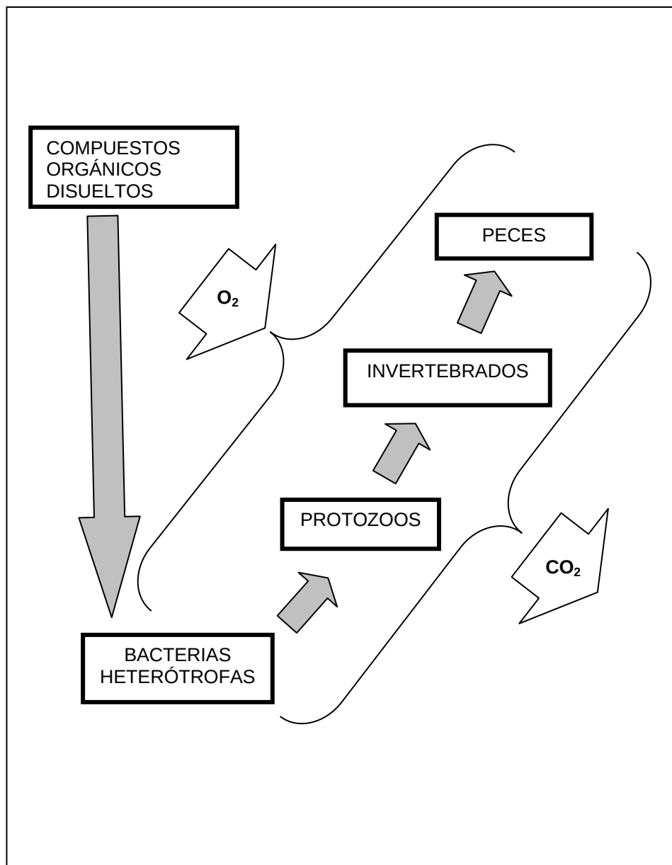
FIGURA 3.9: CADENA TRÓFICA AERÓBICA
