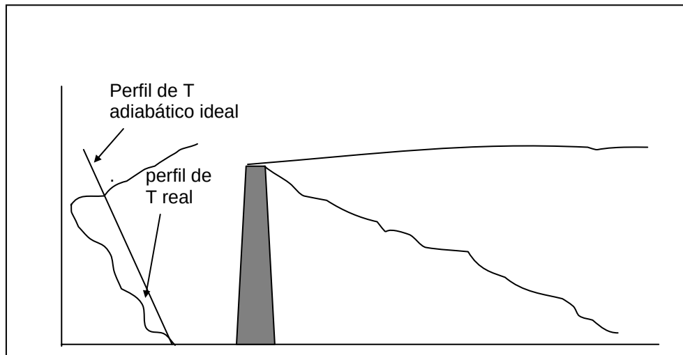
FIGURA 3.5: DISPERSIÓN EN FORMA DE FUMIGACIÓN. INVERSIÓN TÉRMICA QUE IMPIDE ASCENSO DE LA PLUMA. LA PLUMA CAE RÁPIDAMENTE AL SUELO.
