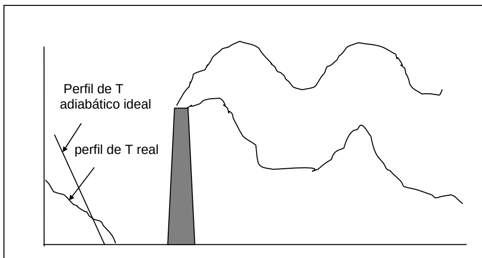
FIGURA 3.2: DISPERSIÓN EN FORMA SERPENTEANTE. ATMÓSFERA INESTABLE, BUENA DISPERSIÓN DE LOS GASES. SIN EMBARGO, LA PLUMA PUEDE TOCAR EL SUELO POR CORTOS INTERVALOS.
