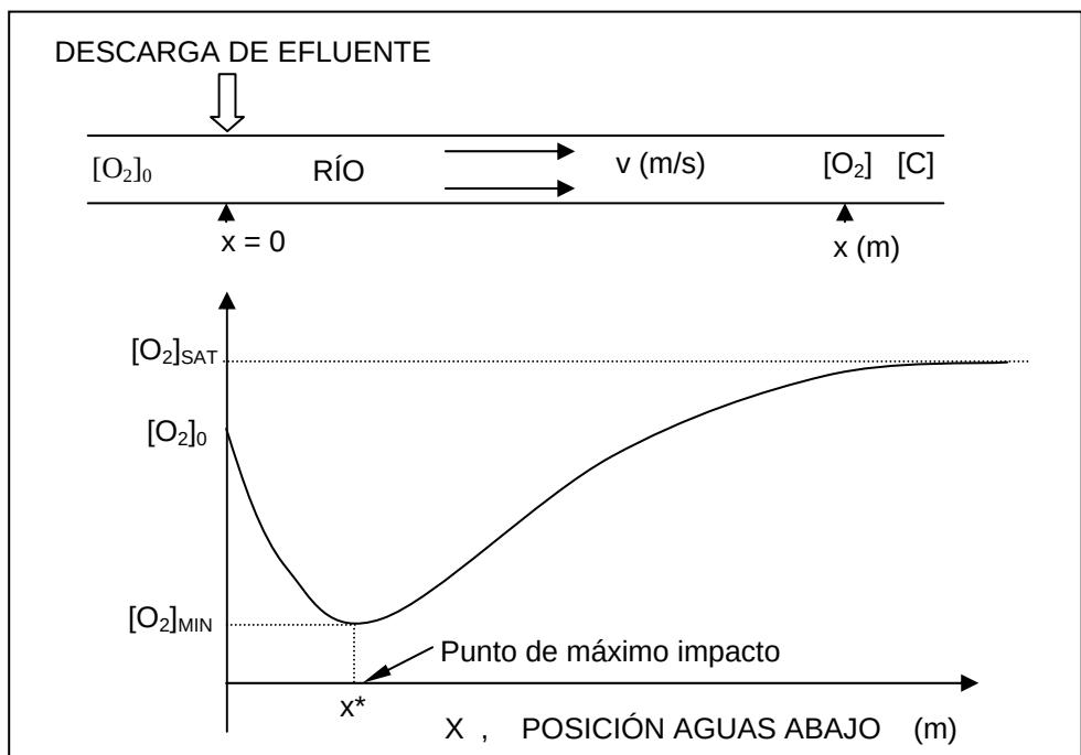
FIGURA 3.11: EFECTO DE UNA DESCARGA DE MATERIAL ORGÁNICO BIODEGRADABLE, SOBRE EL OXÍGENO DISUELTO EN UN RÍO.
