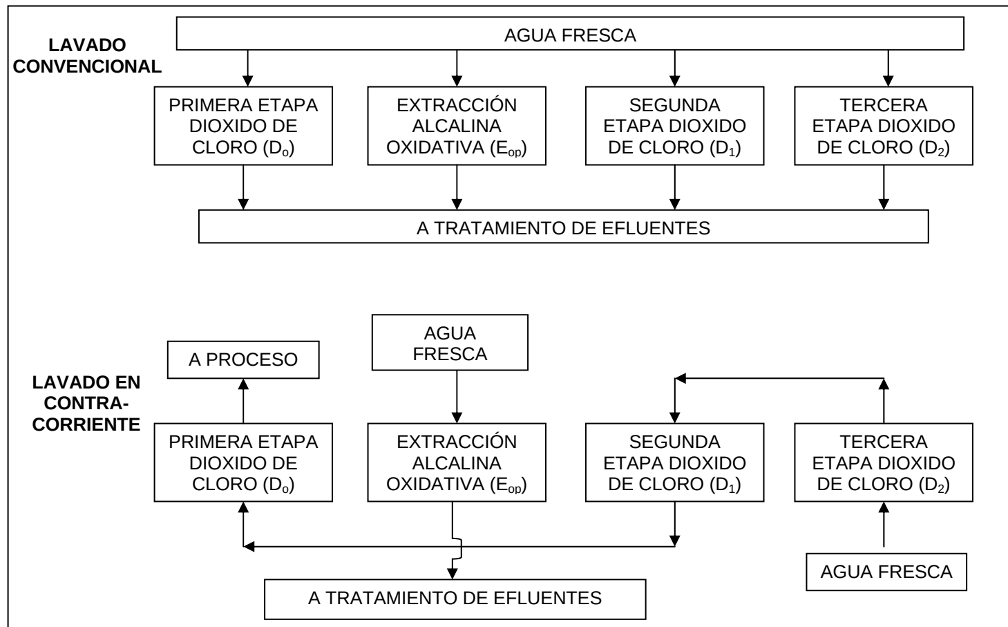
FIGURA 6.7: SISTEMA DE LAVADO DE PULPA CELULOSICA EN SECUENCIA DE BLANQUEO ECF
